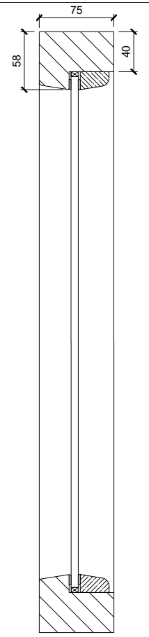
SECTION A-A
